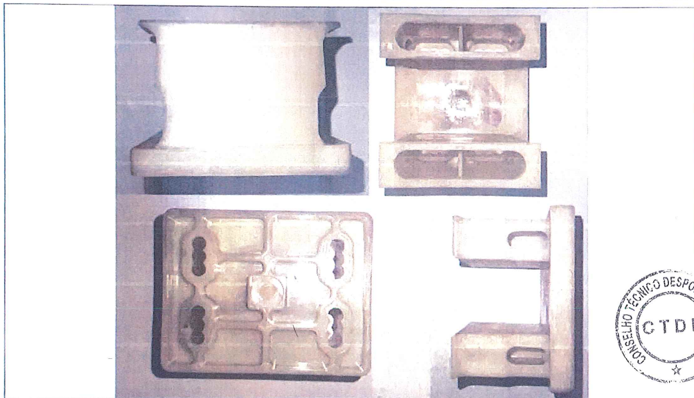
FOTO FRONTAL, SUPERIOR E LATERAL DO BLOCO DE FIXAÇÃO DO PAINEL DIANTEIRO (BICO)
