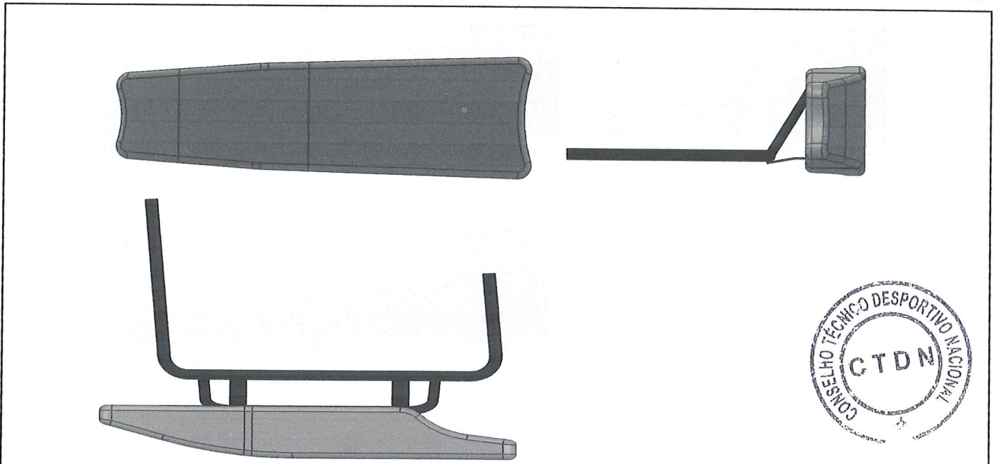
FOTO FRONTAL, SUPERIOR E LATERAL DAS CARENAGENS LATERAIS COM SUPORTES E FIXAÇÕES.
