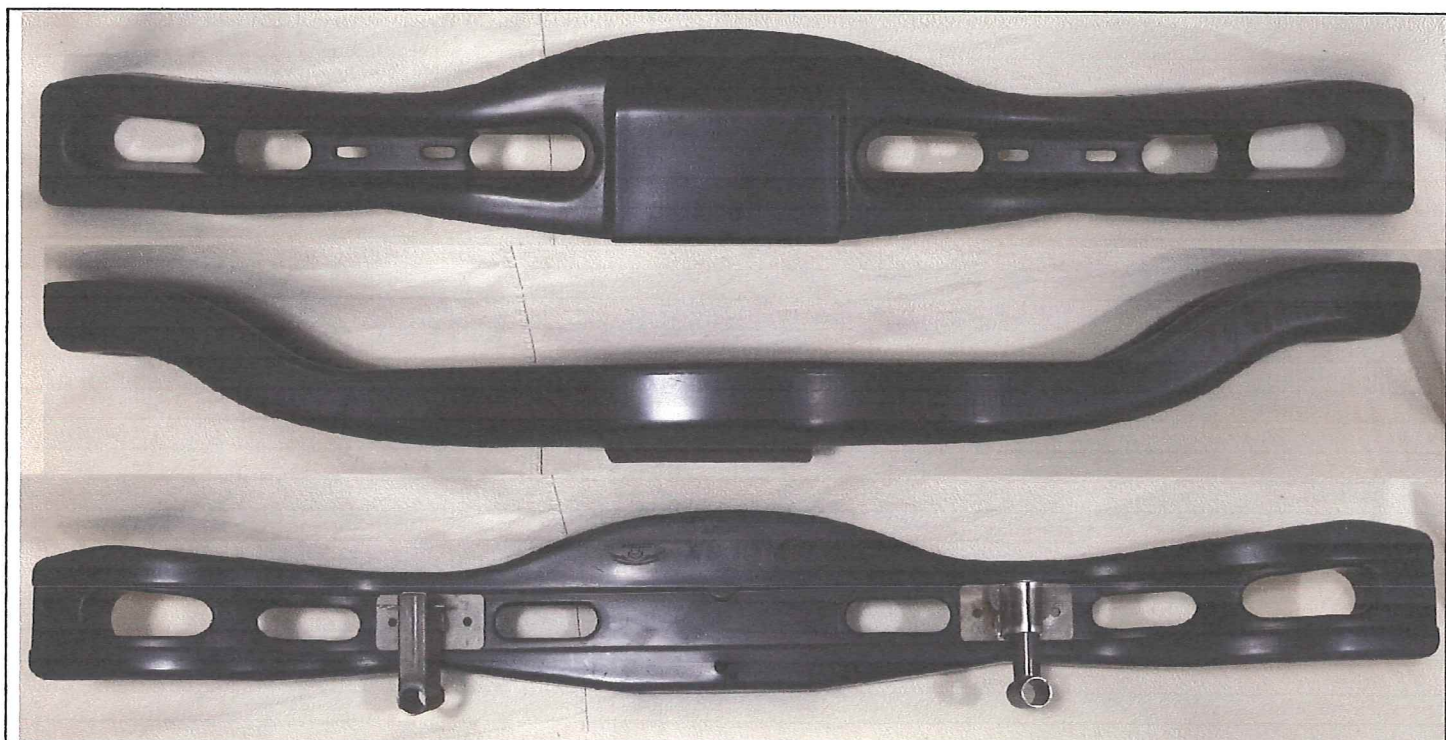
FOTO FRONTAL, SUPERIOR E LATERAL DO PÁRA-CHOQUES TRASEIRO COM SUPORTES E FIXAÇÕES.
