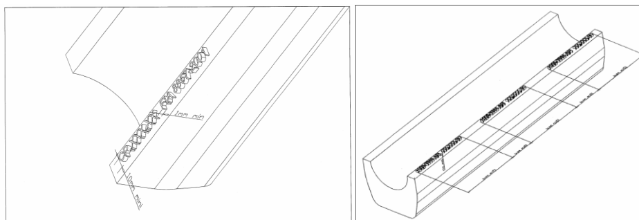
Fig. 22 – Exemplos de marcação e distanciamento dos revestimentos de tubo homologados.
