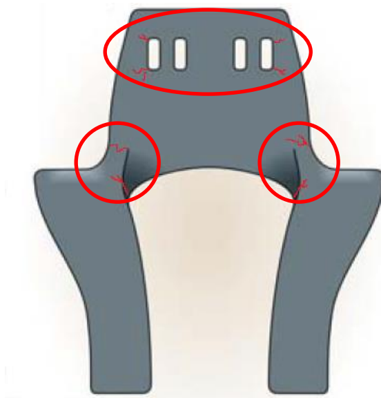
Fig. 19 – Pontos com maior probabilidade de falha no corpo principal do sistema de retenção
