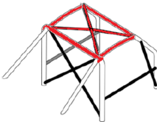
Fig. 21 [Fig FIA Ann J-253-68]: Tubos em que devem ser instaladas as proteções
