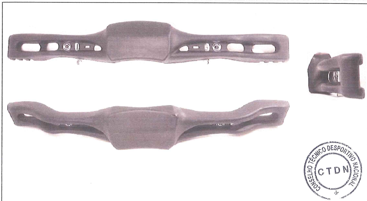
FOTO FRONTAL, SUPERIOR E LATERAL DO PÁRA-CHOQUES TRASEIRO COM SUPORTES E FIXAÇÕES.
